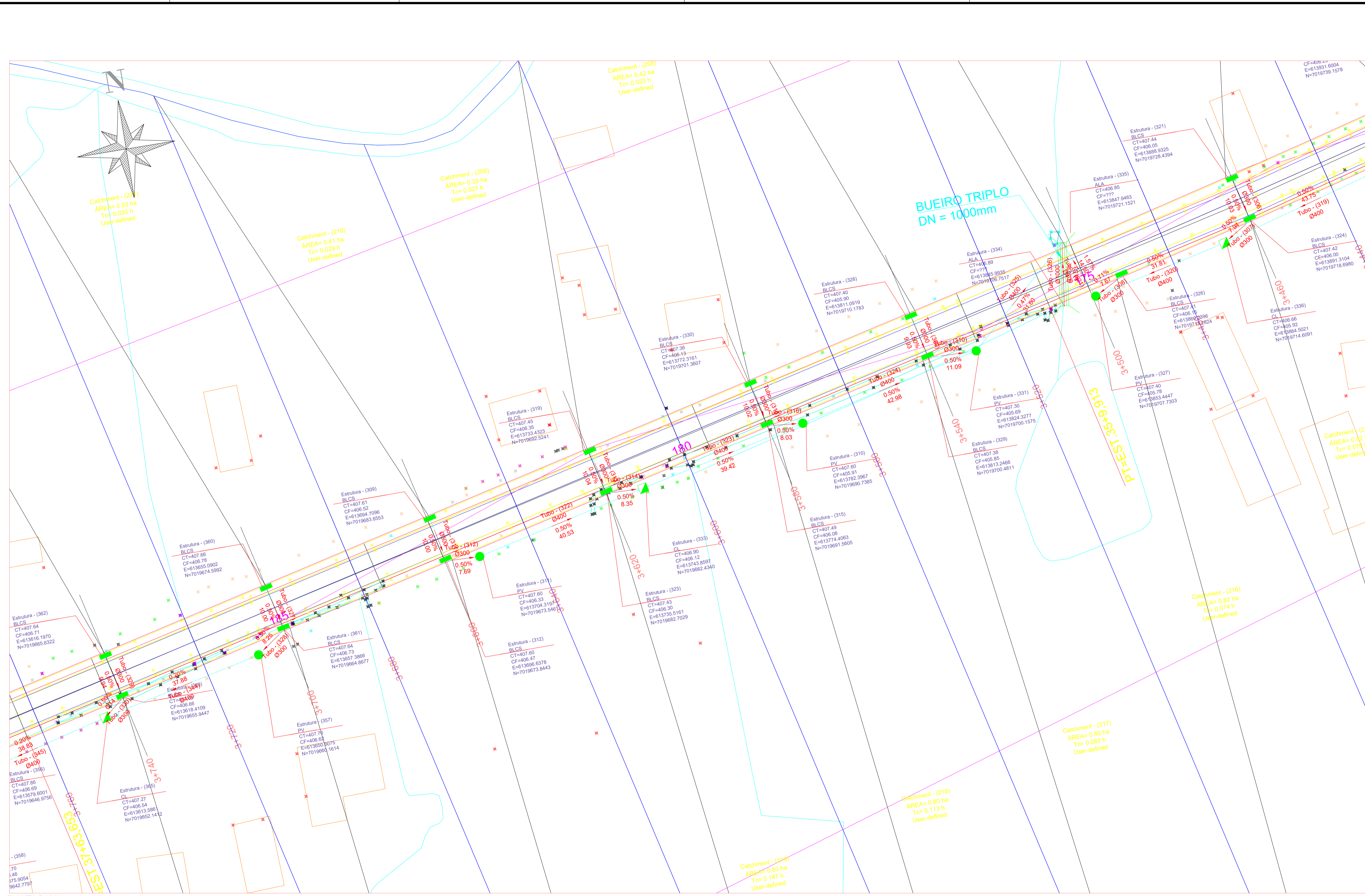
PLANTA BAIXA ESTACA 3+440 A 3+760 ESC: 1/500
