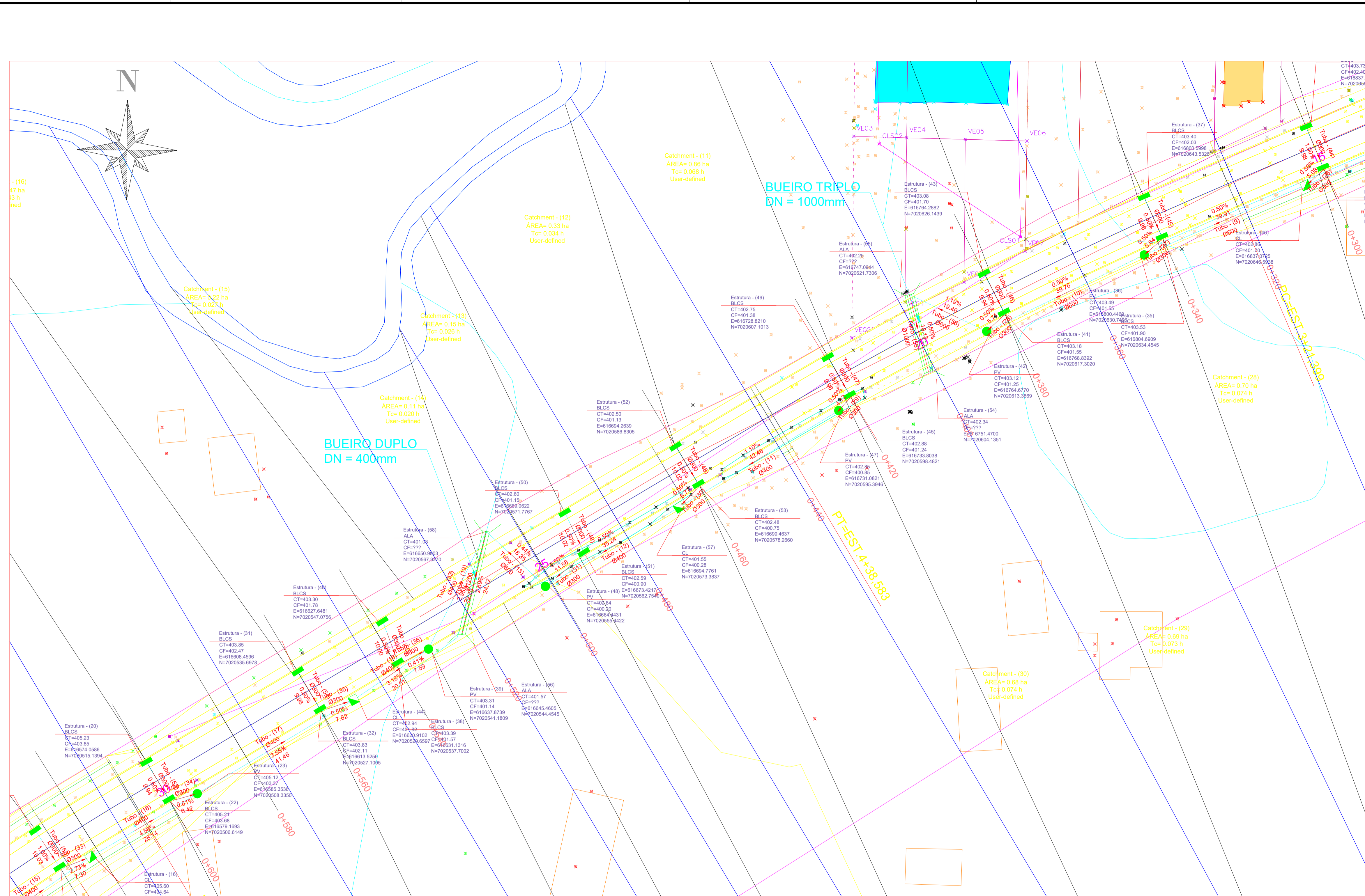
PLANTA BAIXA ESTACA 0+300 A 0+600 ESC: 1/500
