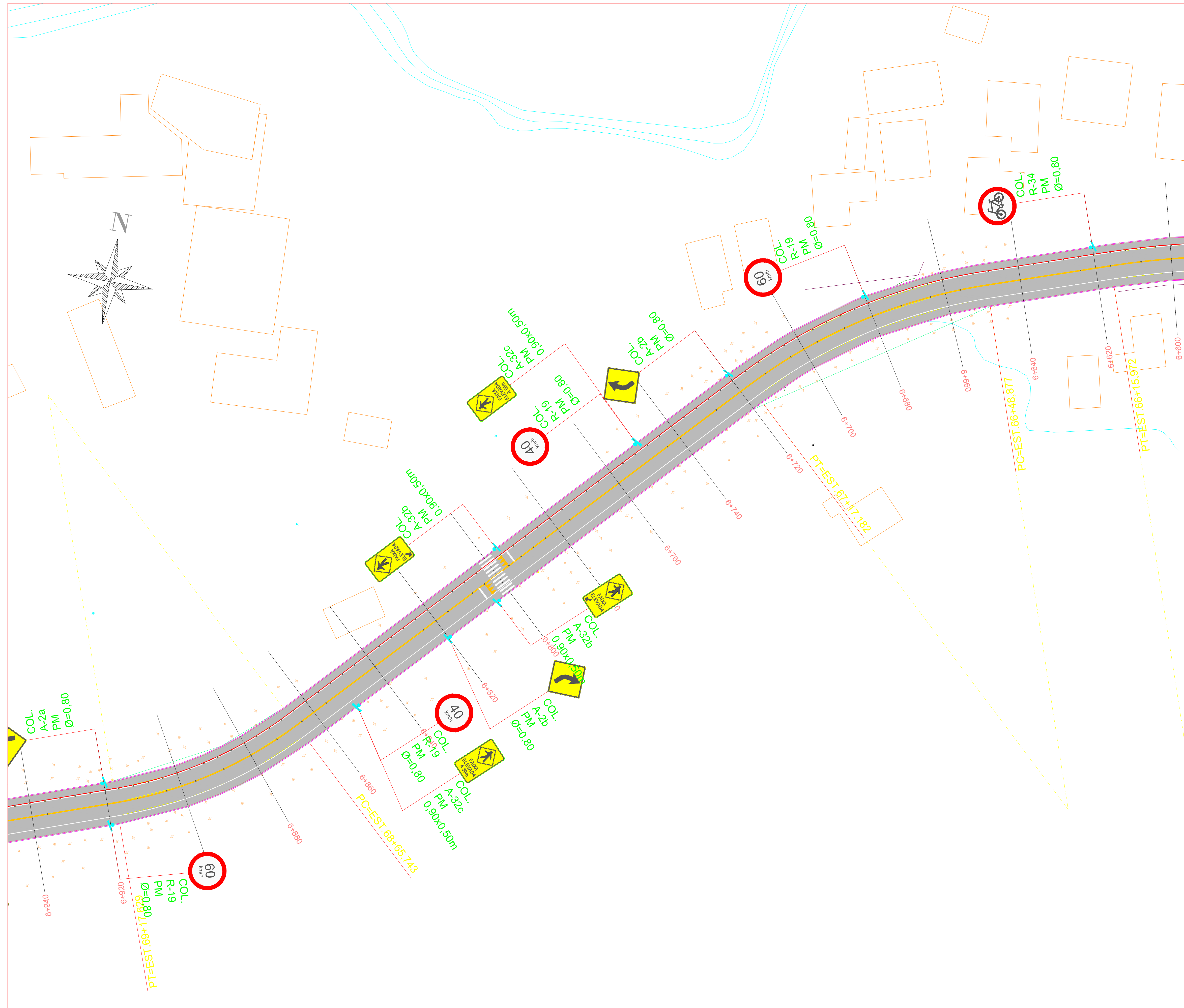
PLANTA BAIXA ESTACA 6+600 A 6+940 ESC: 1/500
